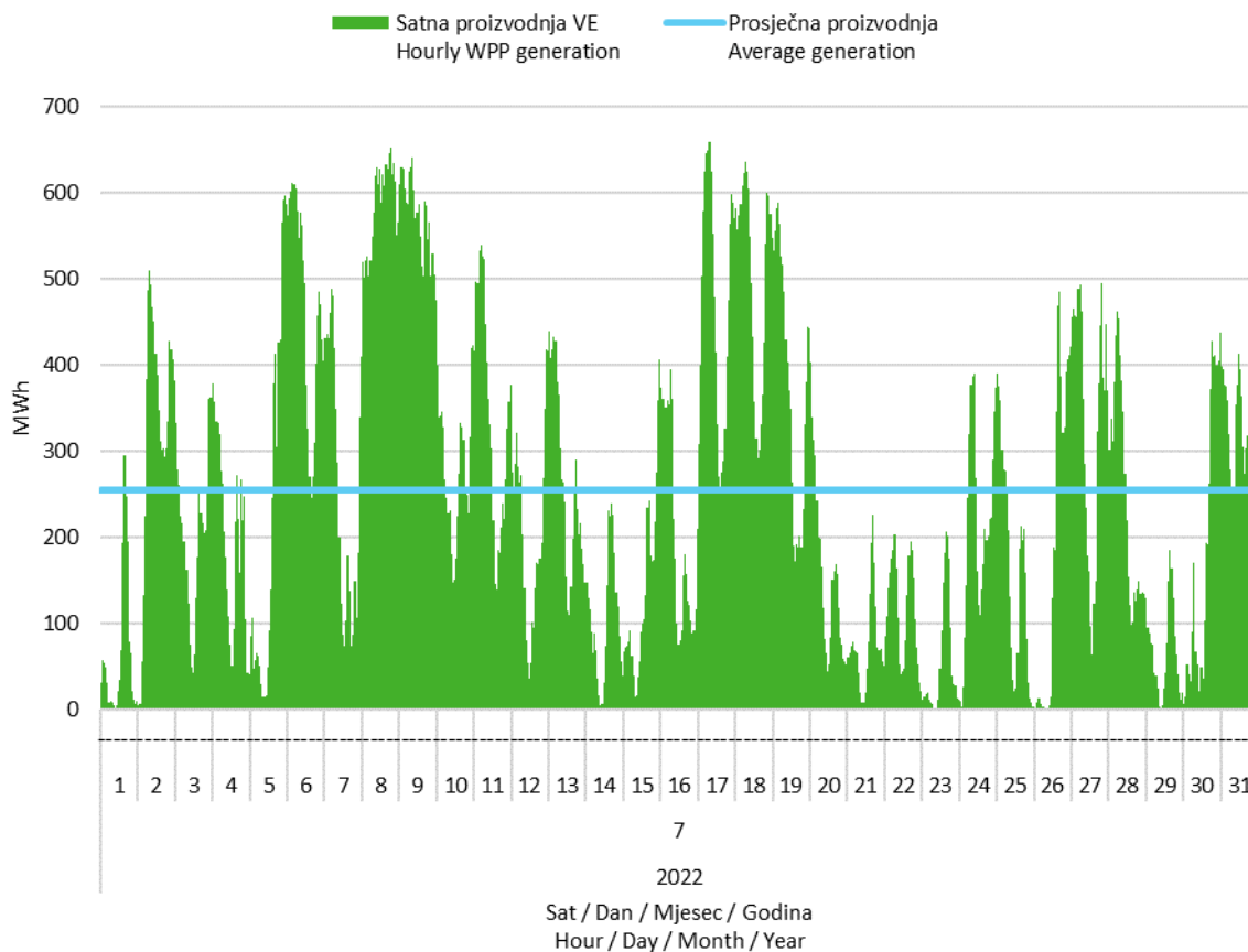
Slika 2 Satna proizvodnja svih vjetroelektrana u srpnju 2022. godine
