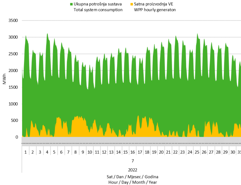
Slika 7 Usporedba satnog dijagrama opterećenja sustava i proizvodnje vjetroelektrana u srpnju 2022. godine
