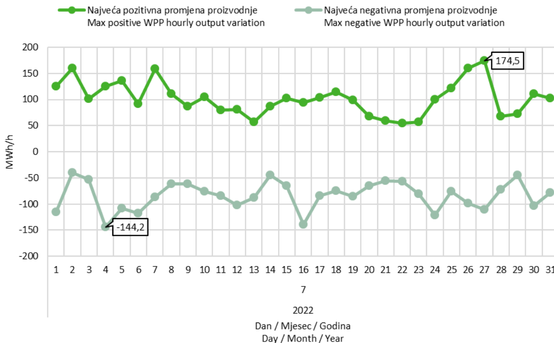
Slika 9 Maksimalna pozitivna i maksimalna negativna promjena satne proizvodnje VE u srpnju 2022. godine
