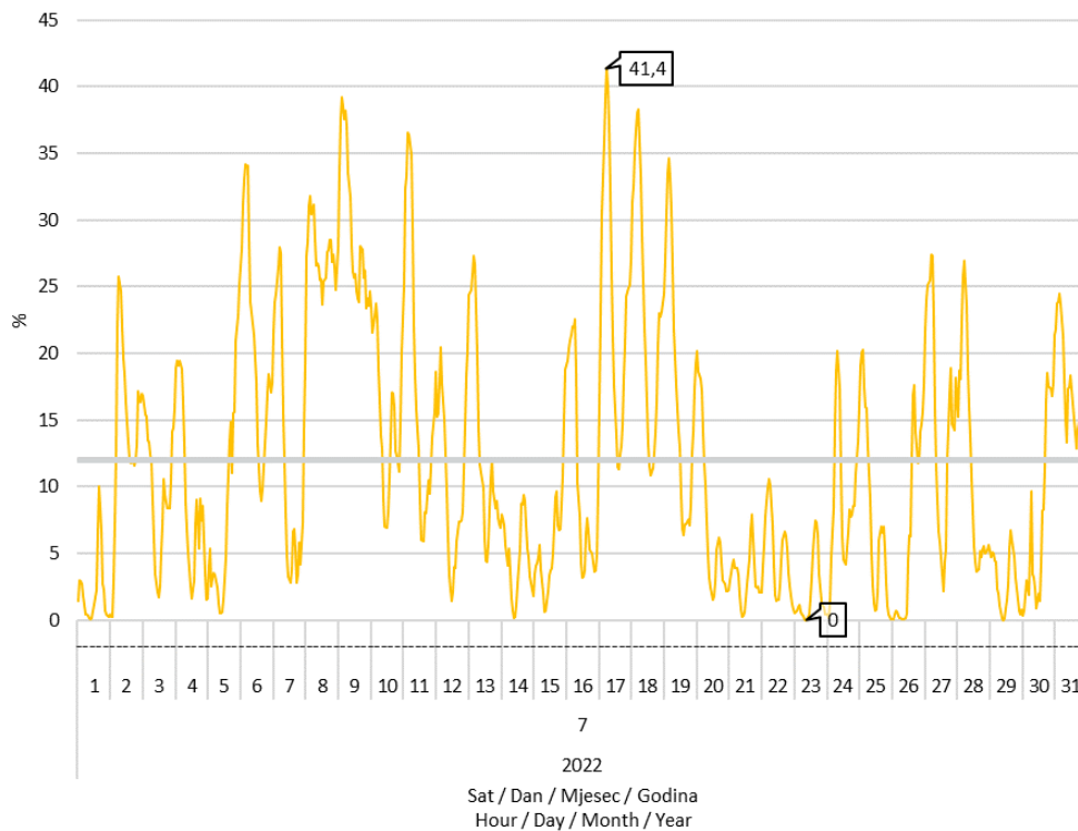
Slika 8 Udio proizvodnje vjetroelektrana u pokrivanju satnog opterećenja elektroenergetskog sustava u srpnju 2022. godine
