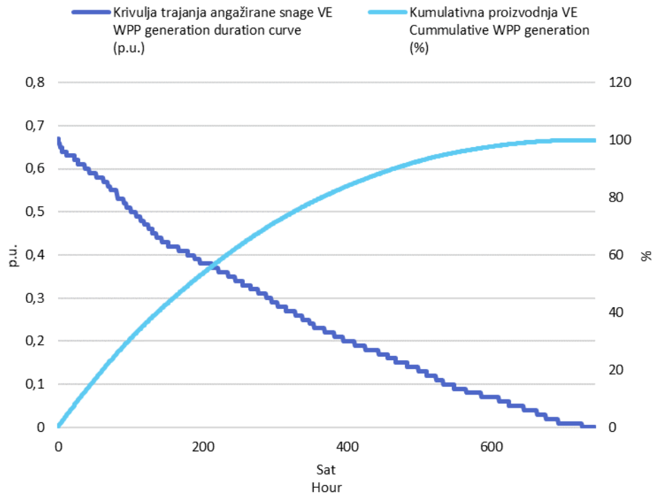
Slika 3 Krivulja trajanja angažirane snage svih VE i kumulativna proizvodnja VE u srpnju 2022. godine u jediničnim vrijednostima
