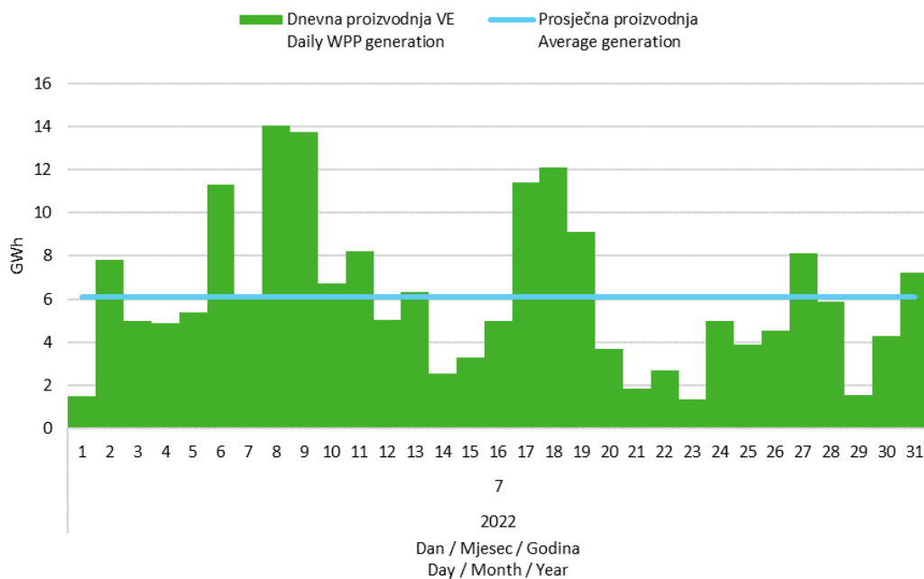
Slika 5 Dnevna proizvodnja svih vjetroelektrana u srpnju 2022. godine Figure 5 Daily generation of all wind power plants in July 2022
