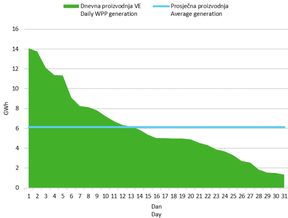
Slika 6 Krivulja trajanja dnevne proizvodnje vjetroelektrana u srpnju 2022. godine
