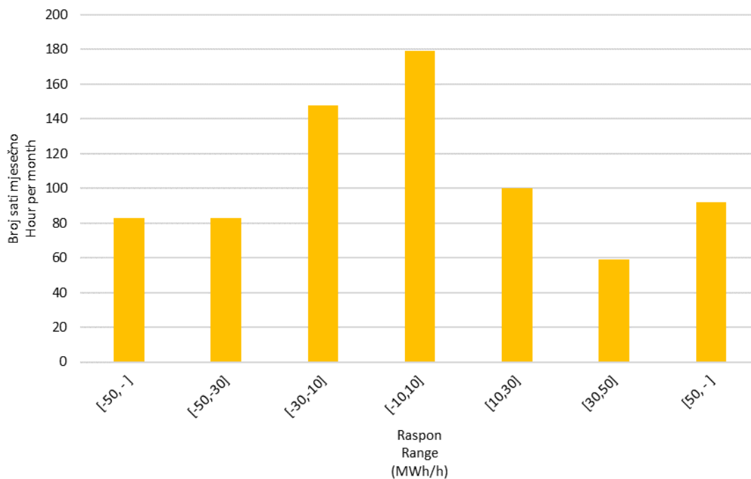
Slika 10 Statistička raspodjela satnih promjena proizvodnje VE u srpnju 2022. godine
